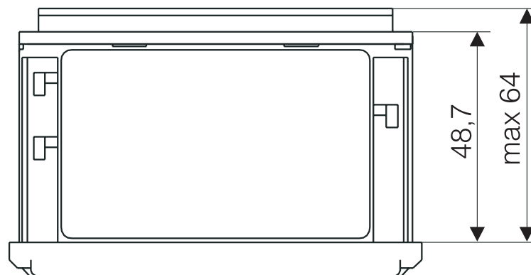
Zchnng. 2. Abmessungen
