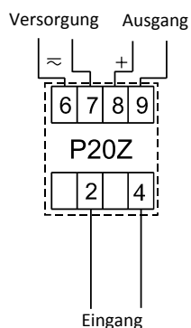
Abb 1. Direkte Messung der Spannung
